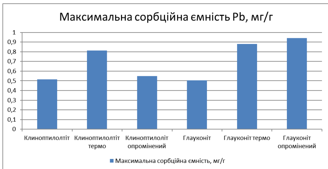
Рис. 4. Максимальна сорбційна ємність зразків по Pb, мг/г
